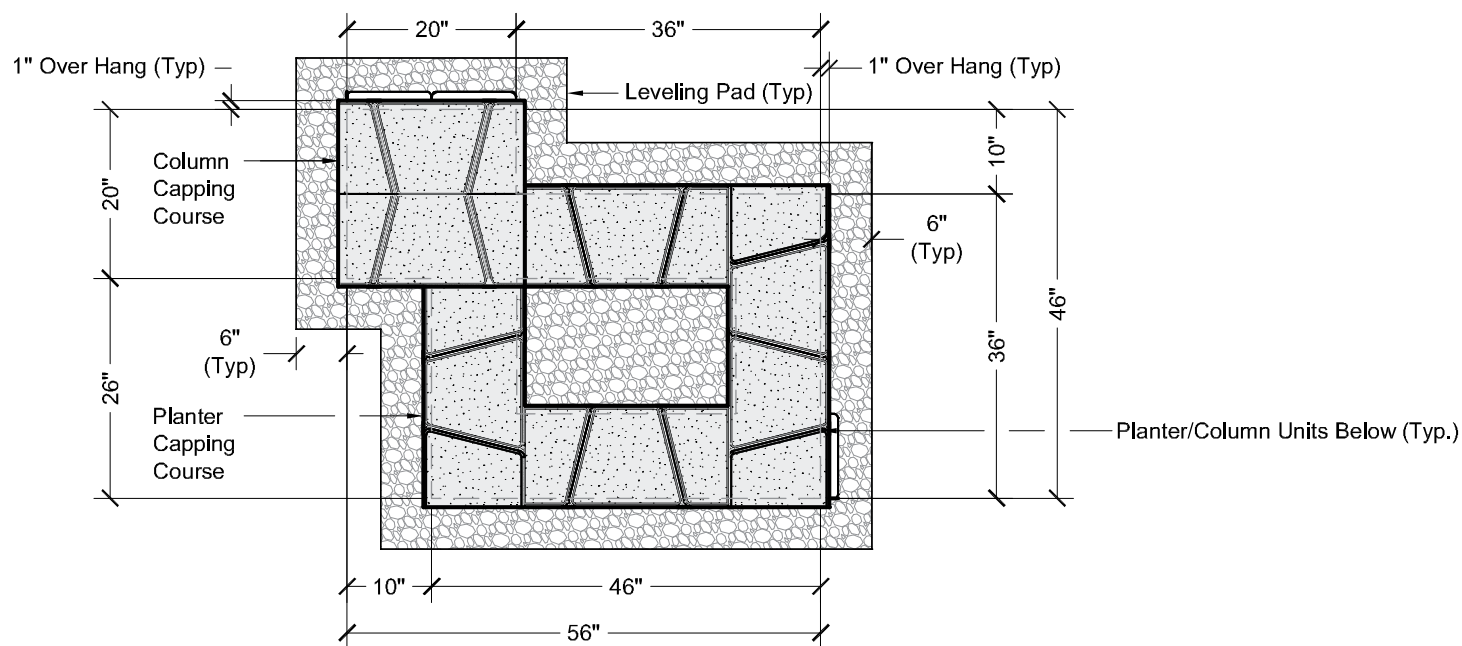
Planter w/Corner Column Plan
